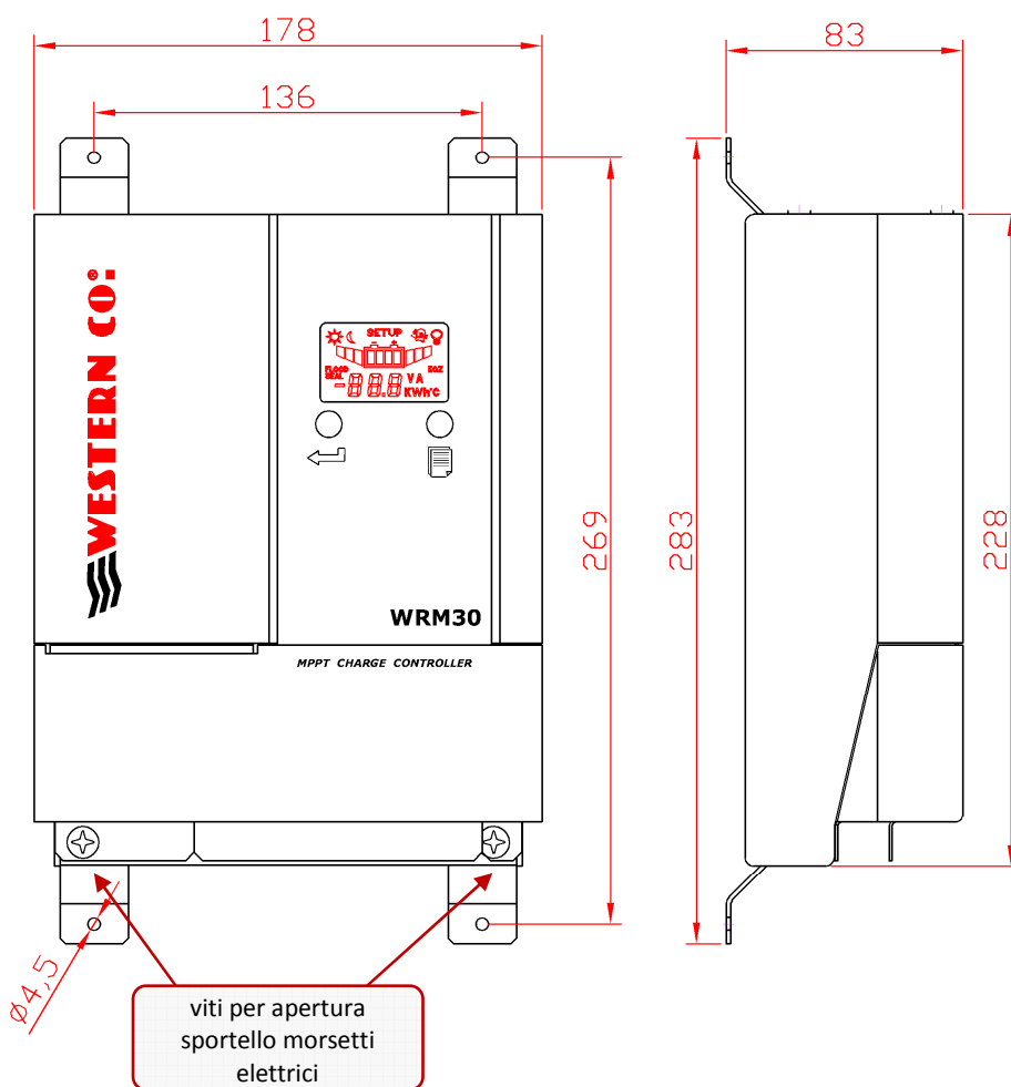
Fig. 4 Dimensioni (mm)
