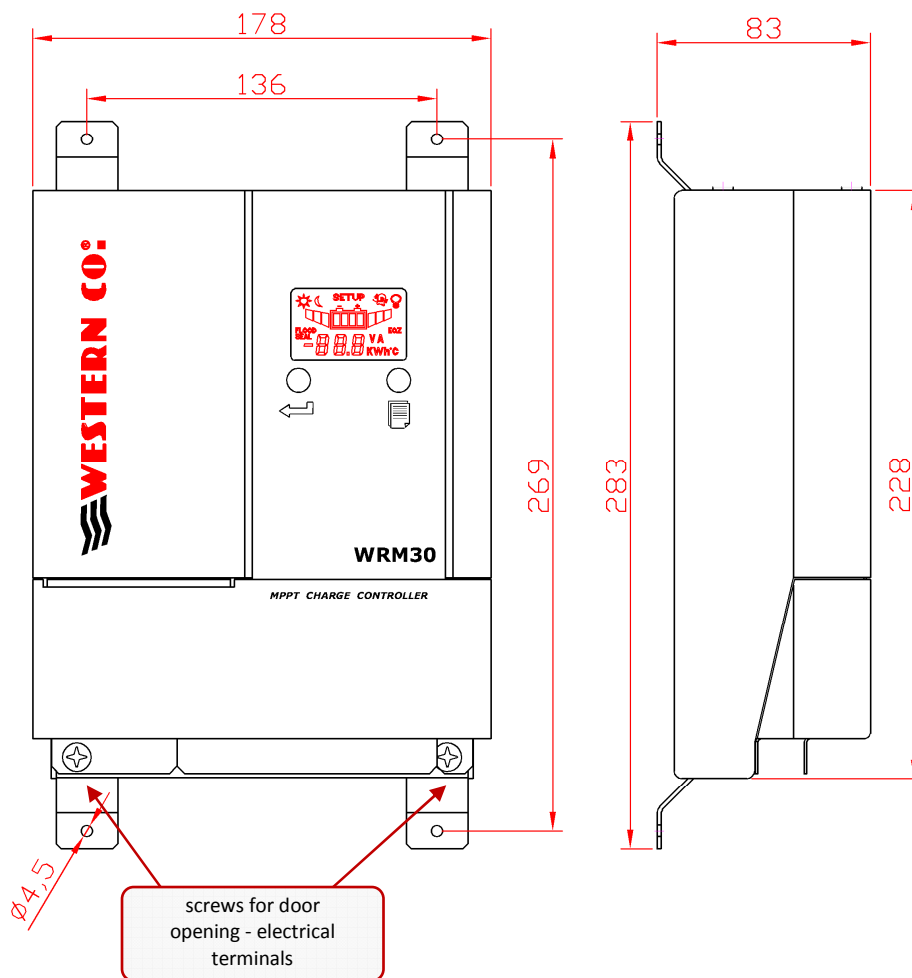
Fig. 4 Dimensions (mm)
